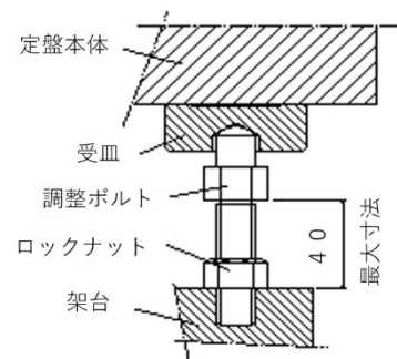
石製精密定盤
